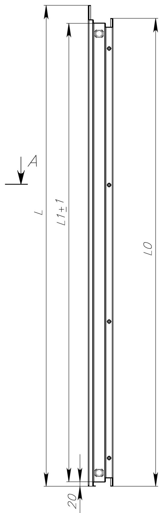
B-B (1 : 10)
