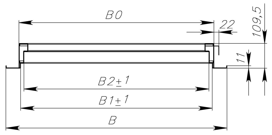
A-A (1 : 10)
